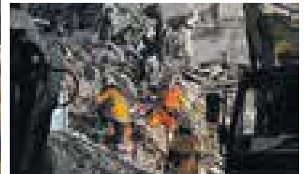
1月29日 紅磡唐樓倒塌事件，由高處俯瞰馬頭圍道唐樓倒塌事故現場。
